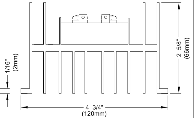
VUE DU BAS / BOTTOM VIEW
